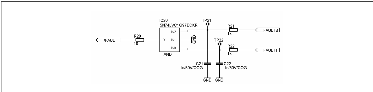
Figure 7 /Fault output
